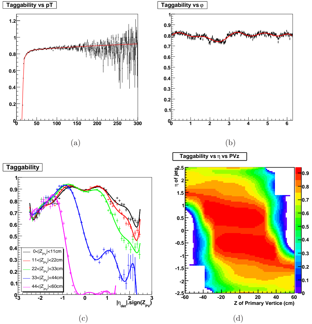
FIG. 5.31 – Étiquetabilité (points noirs) et fonctions d’ajustement de l’étiquetabilité (courbes) selon le p_T (a), le \phi (b) du jet et le couple (\eta, z^{PV}) (c). En (d) est représentée la fonction bidimensionnelle de l’étiquetabilité selon le \eta du jet et le z du vertex primaire.
