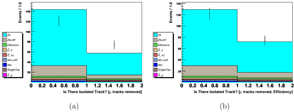
FIG. 5.24 – Booléen “l’événement contient une trace isolée”, les traces des muons étant ôtées des événements, sans (a) et avec (b) correction d’efficacité \epsilon^{isotr k, jet} .
