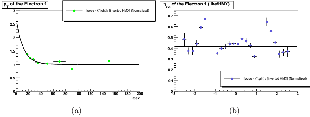
FIG. 4.4 – Rapport \frac{p_T^{EM1}[\text{like-sign}]}{p_T^{EM1}[\text{HMX-2TM}]} du p_T (a) et du \eta_{det} (b) pour l'objet EM dominant lors de la dernière étape de correction. Pour la figure(a) la fonction ajustée est tracée en noir. La ligne noire de la figure (b) représente la moyenne des rapports.
