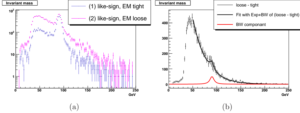
FIG. 4.3 – (a) Masse invariante des lots like-tight (en bleu) et like-loose (en rose). (b) Masse invariante du lot like-loose soustrait par le lot like-tight . La distribution finale est ajustée par une fonction exponentielle plus une Breit-Wigner (en noire). La contribution de la fonction Breit-Wigner est tracée en rouge.
