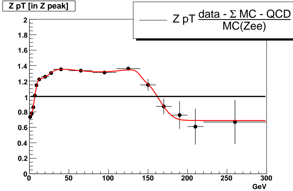
FIG. 4.6 – Rapport des distributions du p_T du Z des données soustraites des bruits de fond différents de Z \rightarrow ee par la simulation Z \rightarrow ee : \frac{\text{data} - \text{QCD}_{\text{corrigé}} - \sum_{\text{différent de } Z \rightarrow ee} \text{MC}_i}{Z \rightarrow ee} . La fonction ajustée (Eq. 4.2) est tracée en rouge, la ligne noire marque la valeur 1, et sert de guide visuel.
