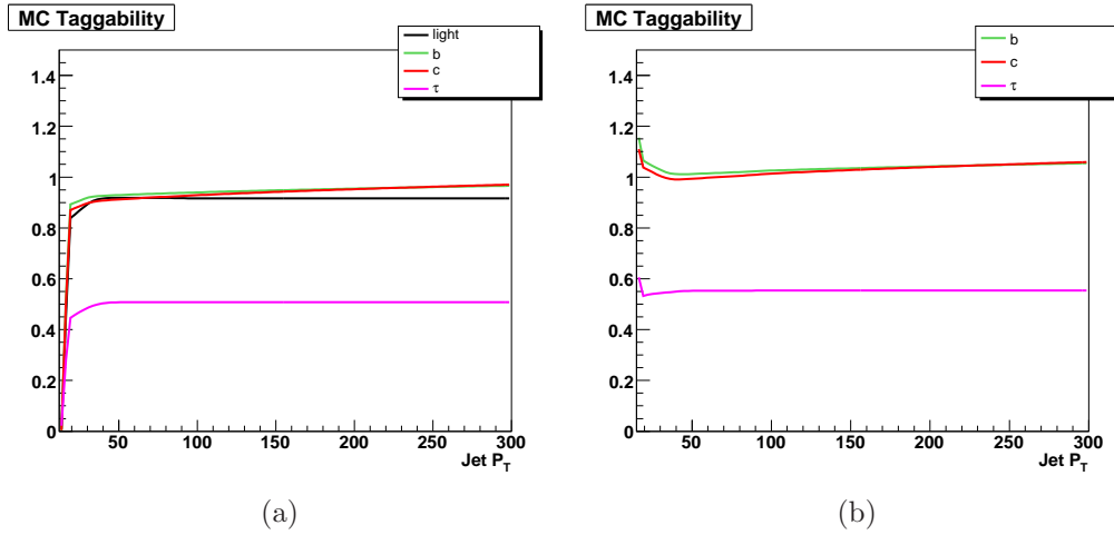
FIG. 5.33 – (a) Étiquetabilités issues de la simulation pour différentes saveurs de jet : saveurs légères (en noir), jets de b (en vert), jets de c (en rouge) et jets de \tau (en rose). (b) Étiquetabilités relatives des saveurs lourdes et des \tau par rapport aux saveurs légères (même code des couleurs qu'en (a)).
