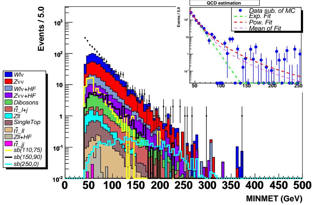
FIG. 5.16 – Distribution de MINMET, toutes les autres coupures étant appliquées. L’excès d’événements dans les données pour de faibles valeurs de MINMET est dû au bruit de fond multijets. L’encadré en haut à droite présente la distribution des données soustraite de celle du bruit de fond électrofaible, avec son ajustement par une loi de puissance (en rouge), une loi exponentielle (en vert), et leur moyenne (en rose) qui donne l’estimation du bruit de fond multijets.
